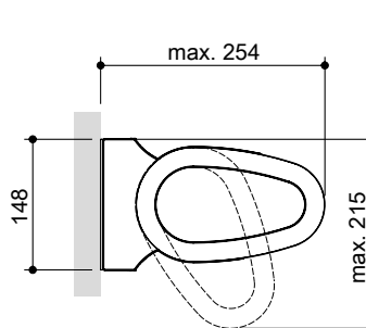
bei Wandmontage 0° - 65°
