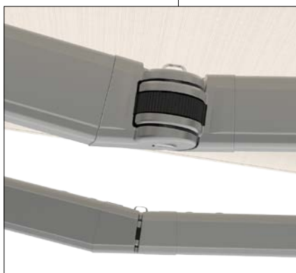
Gelenkarm mit verdeckt liegendem Dyneema® Zugband
